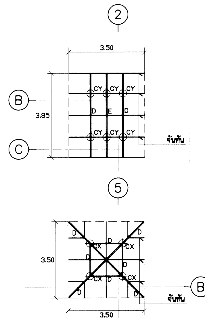
แปลนโครงสร้างหลังคา SCALE 1 : 100
