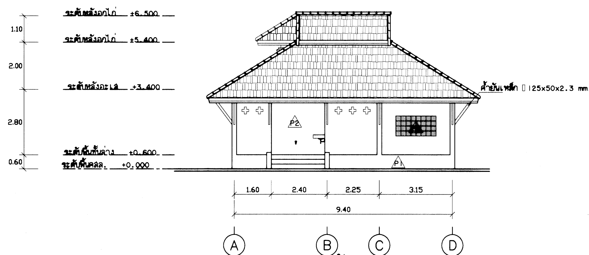
รูปด้าน ④ SCALE 1 : 100
