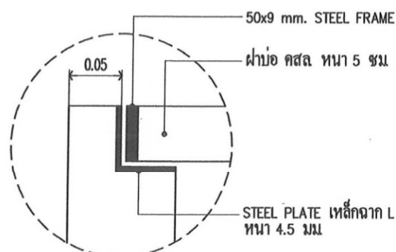
DETAIL เหล็ก PLATE
