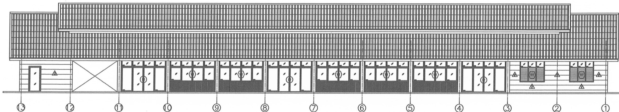
รูปด้าน 3 SCALE A3 = 1:150
