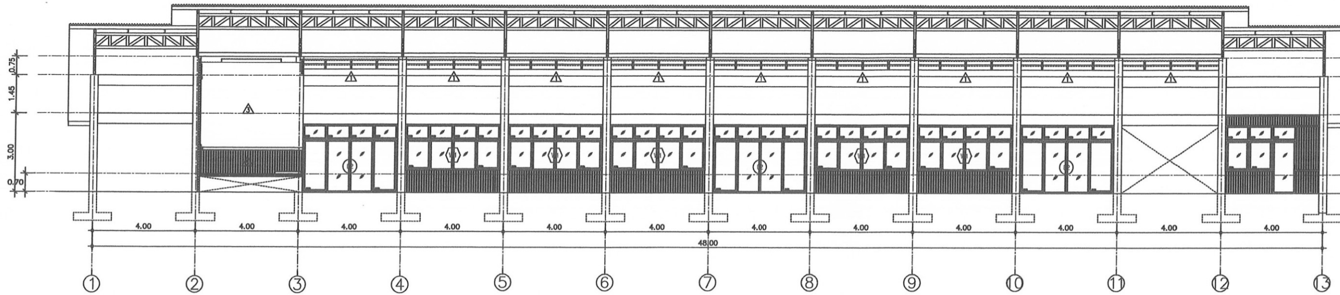
รูปตัด A-A SCALE A3 = 1:150
