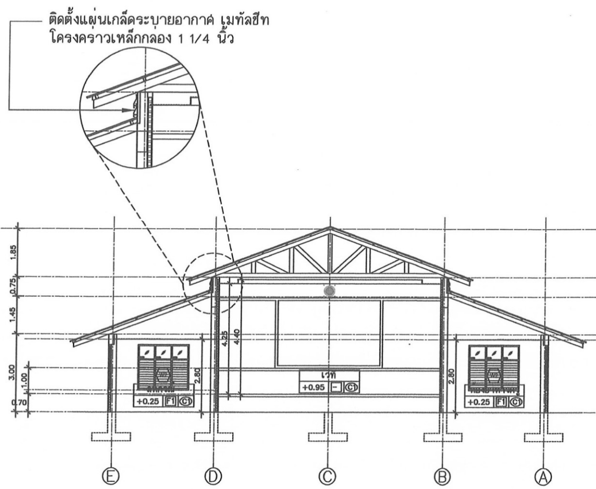
รูปตัด B-B SCALE A3 = 1:150
