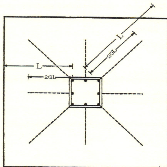
ขยายการตัดเหล็กเสาบนฐานราก
