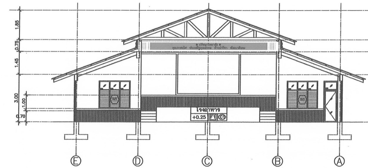
รูปตัด C-C SCALE A3 = 1:150
