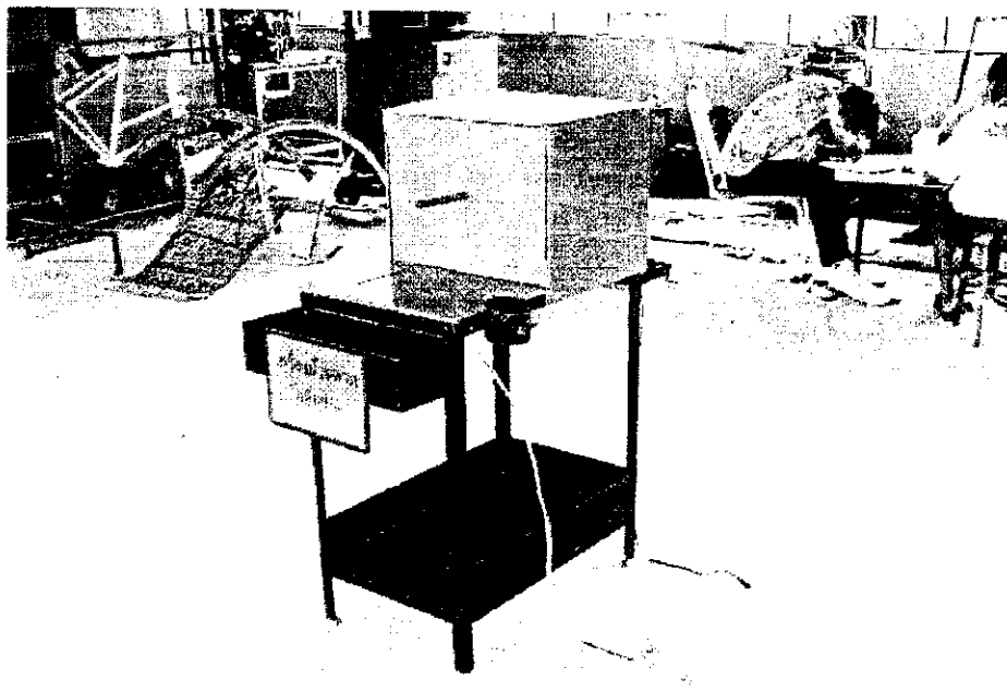
เครื่องมือวัดแรงกดต้นยาง
